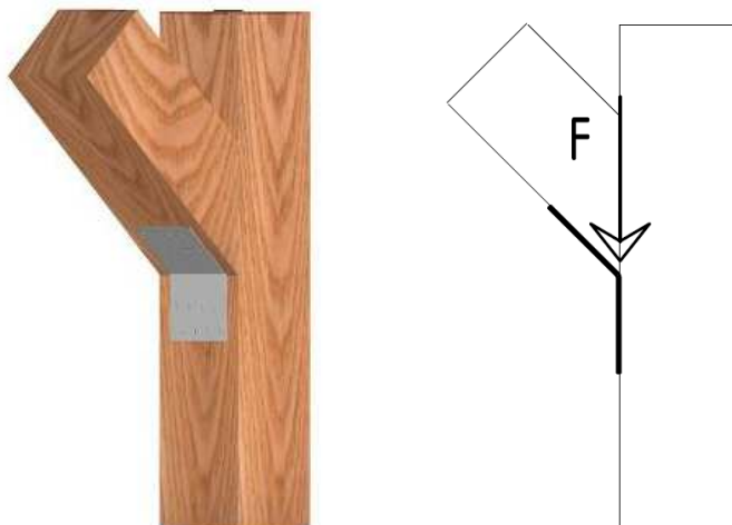
Obr. 1: Směr namáhání 3 ve vztahu ke spojovaným prvkům
