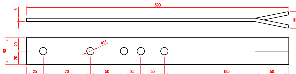
Obr. 1: Kotevní prvek BV-KP 12-06
