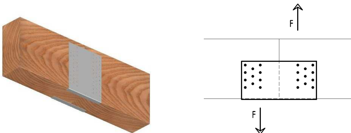
Obr. 1: Směr namáhání 2 ve vztahu ke spojovaným prvkům
